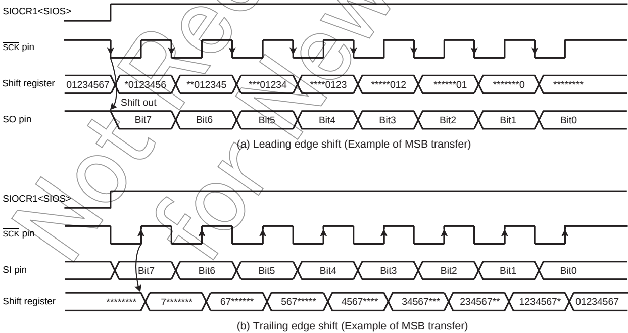
Figure 10-4 Shift Edge
