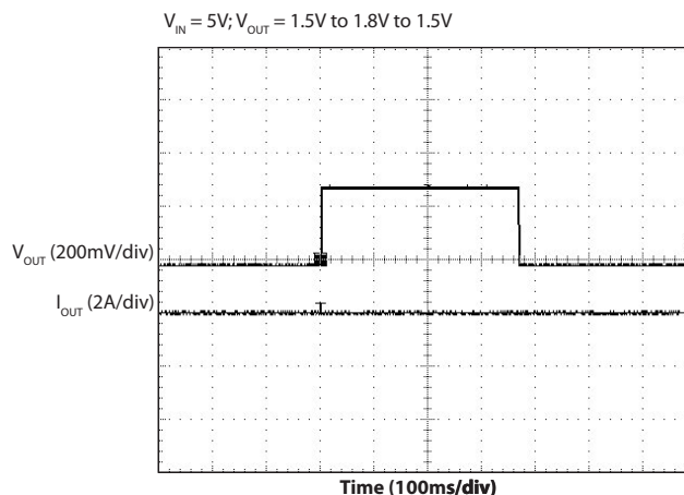
VID Transition — Full Load
