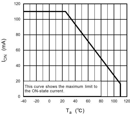
Fig. 12.1.2 I_{ON} - T_a
