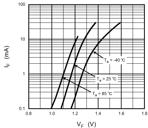
Fig. 12.1.3 I_F - V_F
