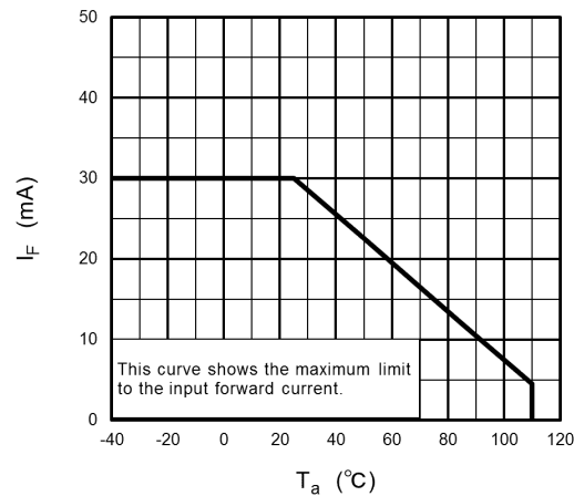
Fig. 12.1.1 I_F - T_a
