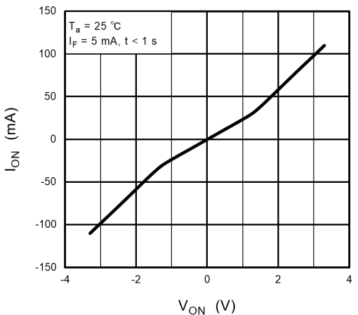
Fig. 12.1.4 I_{ON} - V_{ON}
