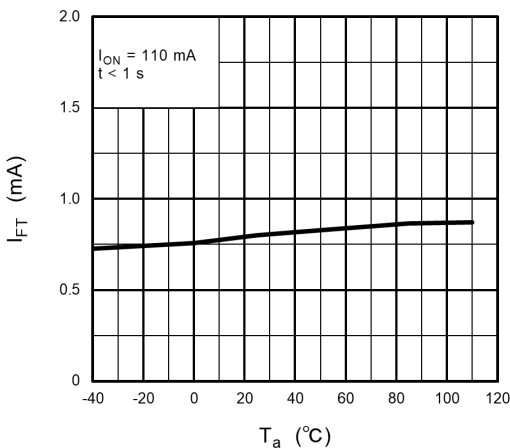
Fig. 12.1.6 I_{FT} - T_a
