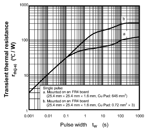
Fig. 8.11 r_{th(j-a)} - t_w
