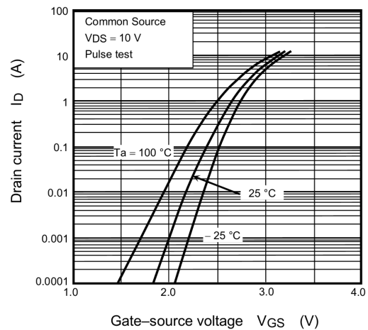
Fig. 8.2 I_D - V_{GS}
