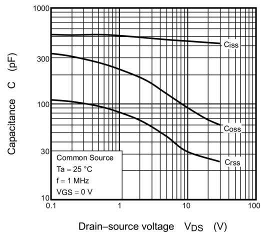
Fig. 8.8 C - V_{DS}
