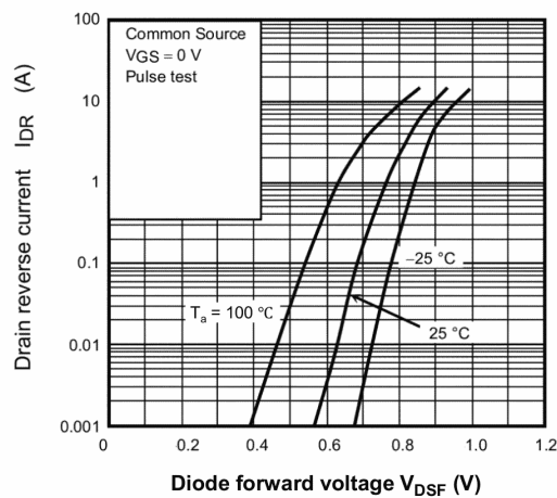
Fig. 8.7 I_{DR} - V_{DSF}
