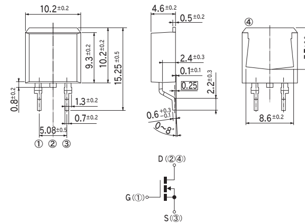
H3 Package: TO-263AB-1
