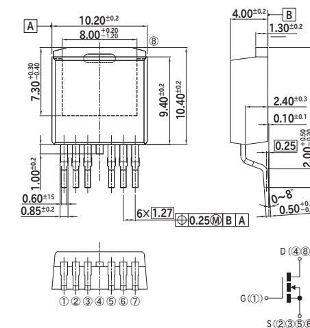
H7 Package: TO-263SC
