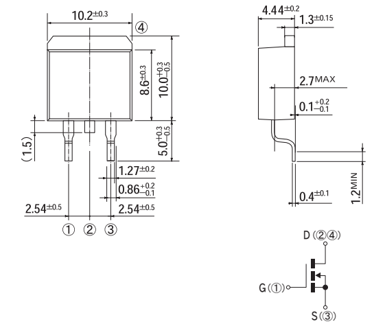
H4 Package: TO-263AB
