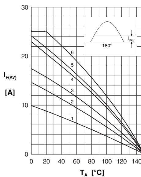
Fig. 4: Load diagramm
