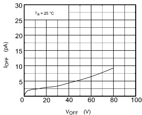
Fig. 12.1.9 I_{OFF} - V_{OFF}
