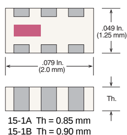
Case 15-1 (EIA 0805 / 1212)
