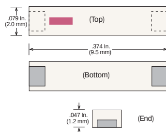
Case 45-1
