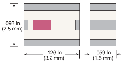
Case 41-1 (EIA 1210 / 3225)
