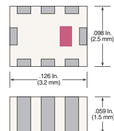
Case 41-2 (EIA 1210 / 3225)
