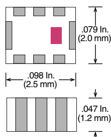
Case 15-2 (EIA 0805 / 1212)
