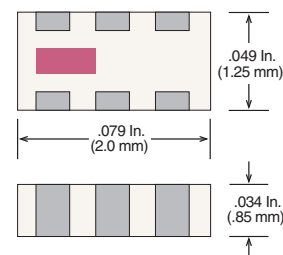
Case 15-1 (EIA 0805 / 1212)
