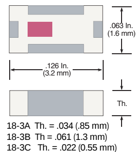
Case 18-3 (EIA 1206 / 3216)
