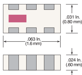
Case 14-1 (EIA 0603/ 1608)
