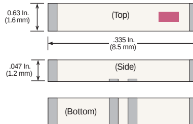
Case 46-1
