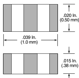
Case 07-1 (EIA 0402/ 1005)
