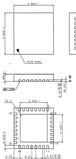
VQFN032V5050 (Unit:mm)
