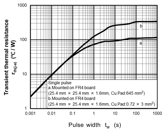
Fig. 8.11 r_{th(j-a)} - t_w
