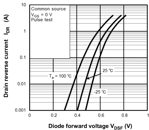
Fig. 8.7 I_{DR} - V_{DSF}
