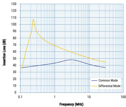
GTX-3500-Y473
