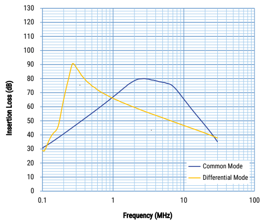
GTX-3600-Y683
