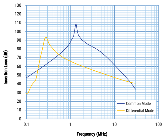
GTX-3600-Y474
