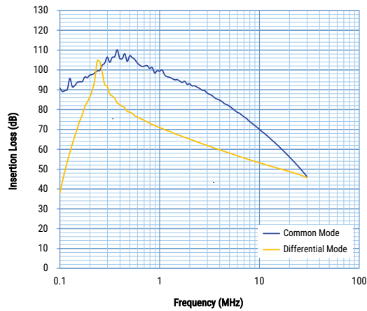
GTX-3400-Y474
