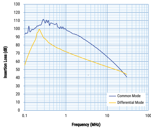
GTX-3300-Y474
