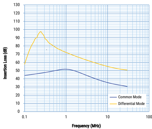
GTX-3300-Y473
