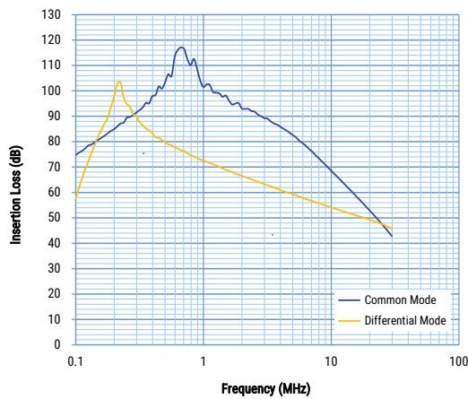
GTX-3300-Y104
