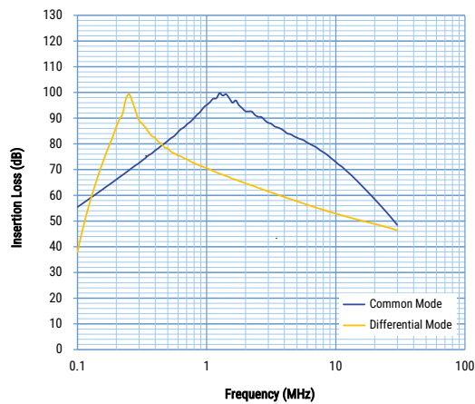
GTX-3400-Y683
