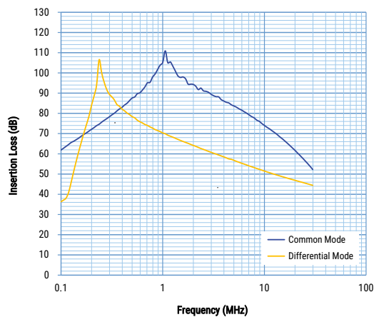
GTX-3500-Y474
