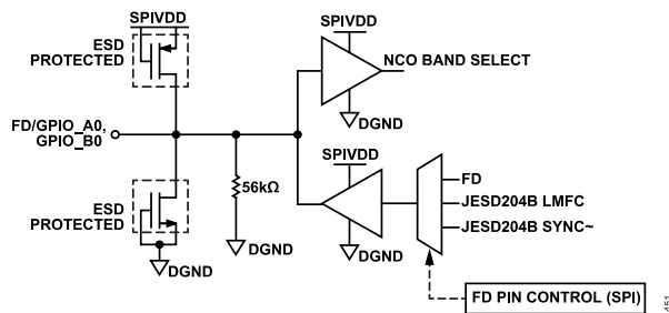
Figure 51. FD/GPIO_A0, GPIO_B0
