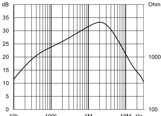
RT 8132
