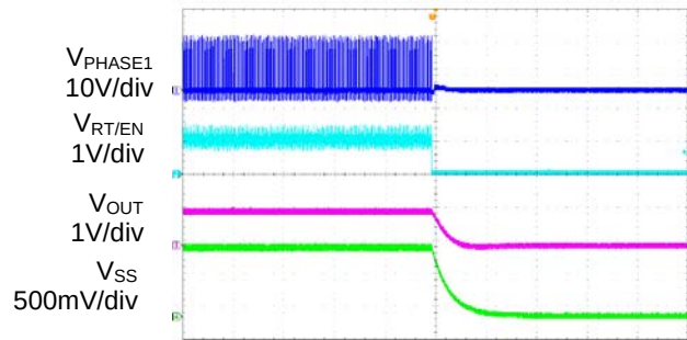
EN Off Waveform
