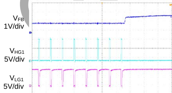
OVP Function
