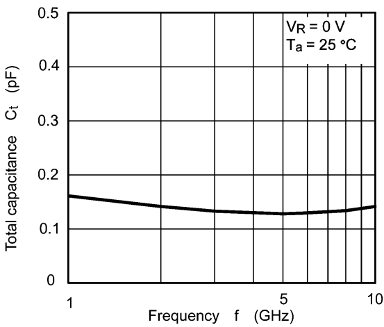
Fig. 9.4 C_t - f
