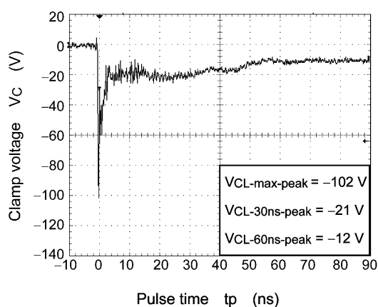
Fig. 6.1.2 -8 kV
