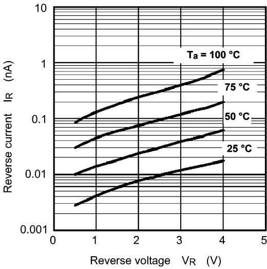
Fig. 9.2 I_R - V_R
