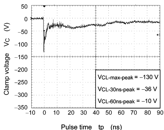
Fig. 6.1.4 -15 kV
