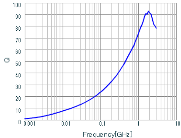
LQW15AN10NJ8Z Q.
