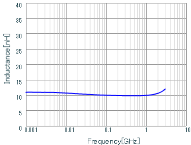
LQW15AN10NJ8Z L.
