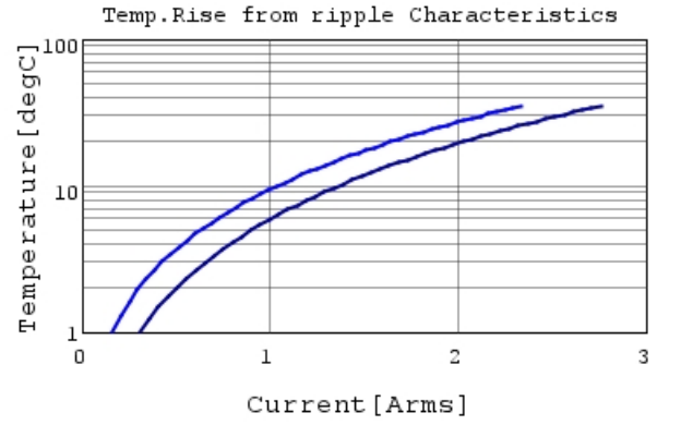
GRM188R71A105KA61 Temp.rise — 500kHz —
