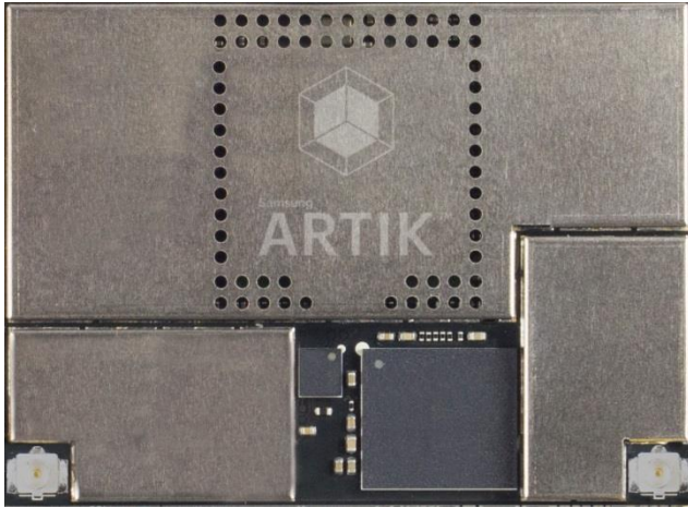
ARTIK 710 Module Top View
