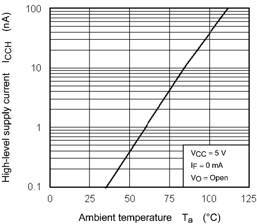
Fig. 12.2.4 I_{CCH} - T_a
