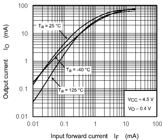
Fig. 12.2.7 I_O - I_F
