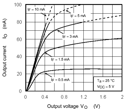
Fig. 12.2.11 I_O - V_O
