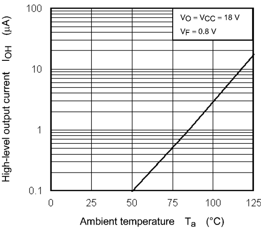
Fig. 12.2.3 I_{OH} - T_a
