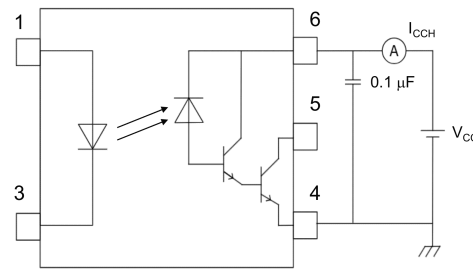
Fig. 12.1.2 I_{CCH} Test Circuit
