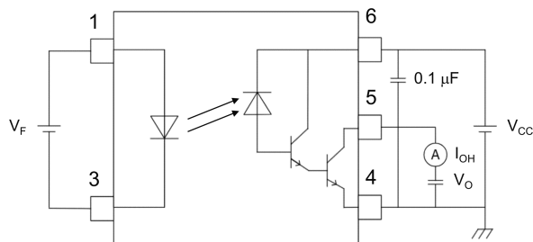
Fig. 12.1.1 I_{OH} Test Circuit
