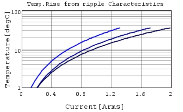
GCM155C71A474ME36 Temp.rise — 200kHz
