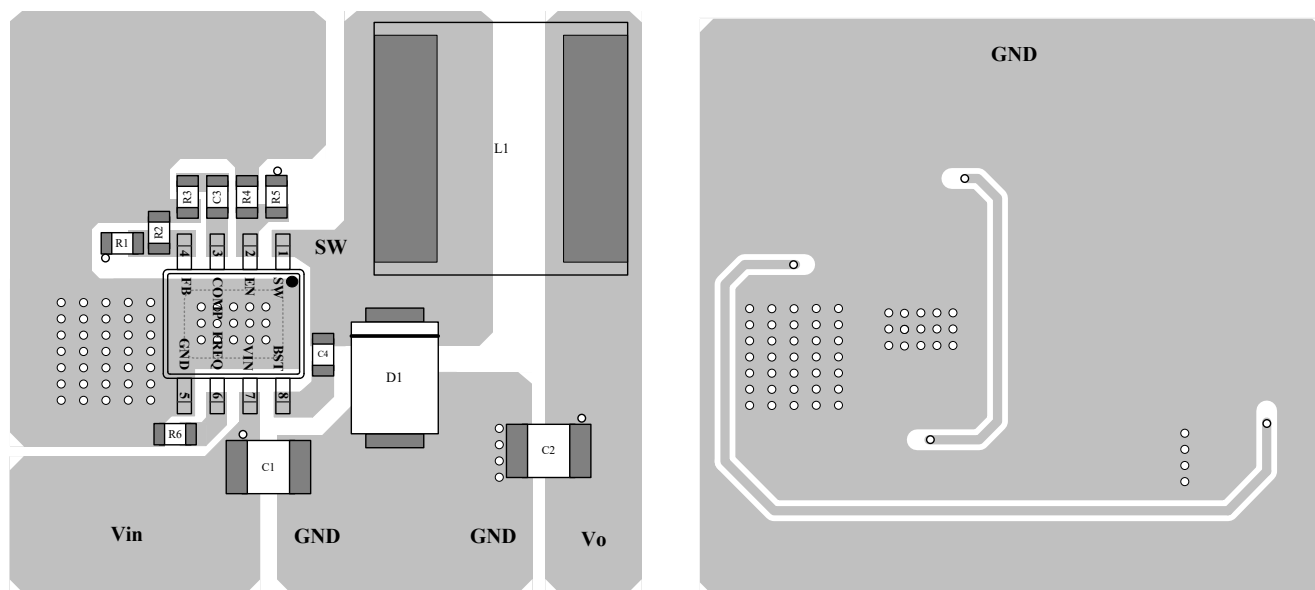
TOP Layer
