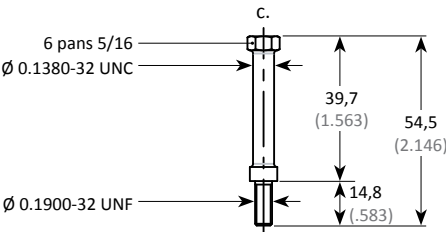
7 Vis à colonnette Pillar bolt
