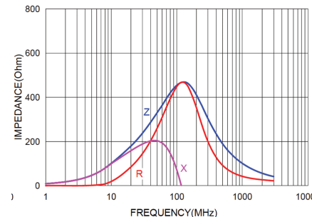
NCB-HD1206B471TR400F NCB-HD1206B471TR400QYF
