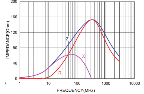
NCB-HD1206B121TR600F NCB-HD1206B121TR600QYF
