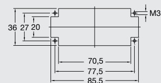
Montageausschnitt Panel cut-out
