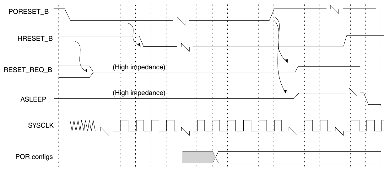
Figure 3-3. POR sequence
