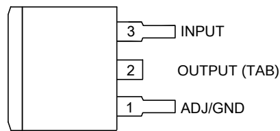
TO263-2
