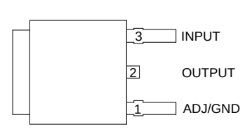
TO252-2 (5)
