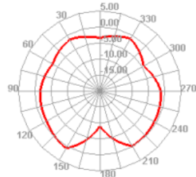
960.000MHz E2
