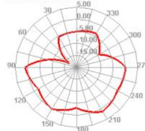
1850.000MHz E2
