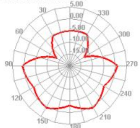
1850.000MHz E1
