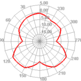
1700.000MHz E1
