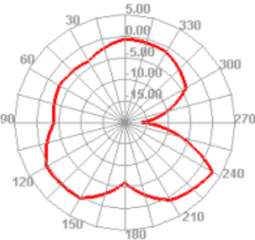
1700.000MHz E2
