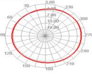
2100.000MHz E2
