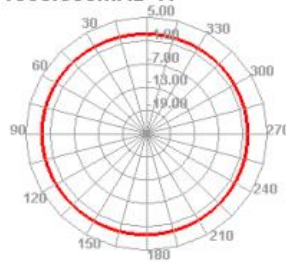
1850.000MHz H
