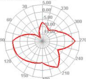
2100.000MHz E2
