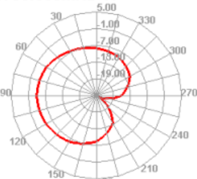
1700.000MHz H
