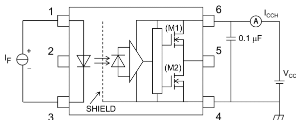
Fig. 13.1.5 I_{CCH} Test Circuit
