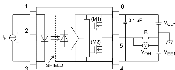
Fig. 13.1.3 V_{OH} Test Circuit
