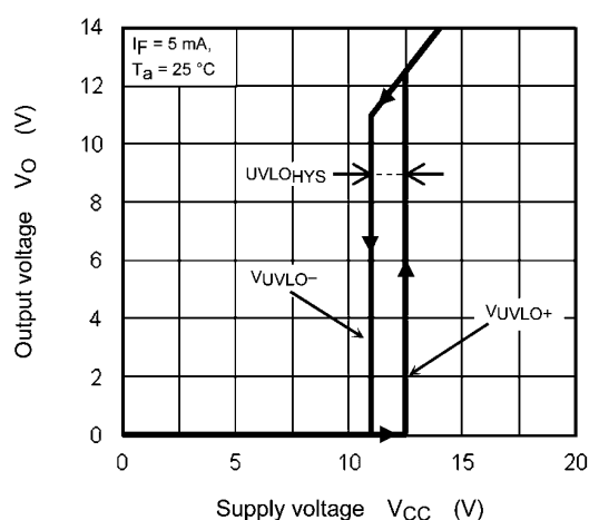
Fig. 13.2.11 V_O(V_{UVLO}) - V_{CC}
