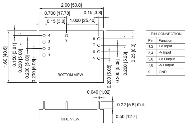
FM20-100 Package
