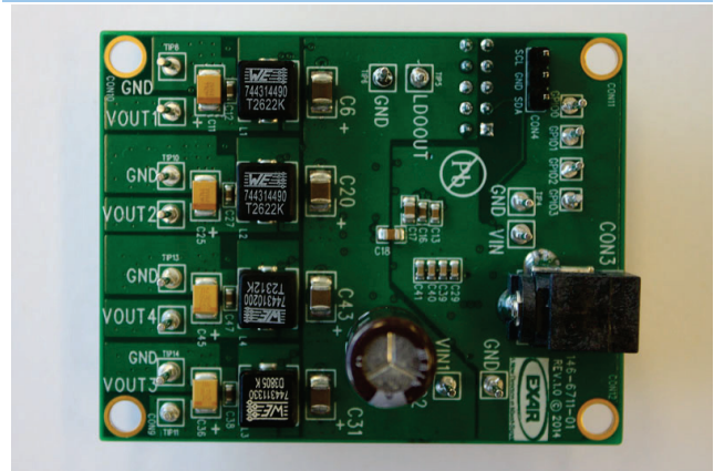
XRP7714EVB-DEMO-3
