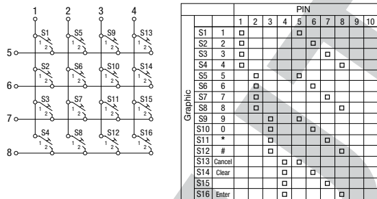
16 key piezo keypad
