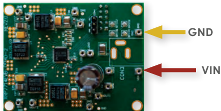
XRP7714EVB-DEMO-2
