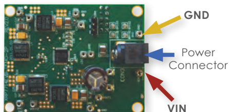
XRP7714EVB-DEMO-2P
