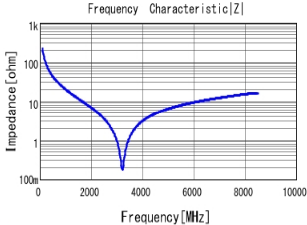
■ GCQ1555C1H7R1DB01 |Z| DC0V, 25degC
