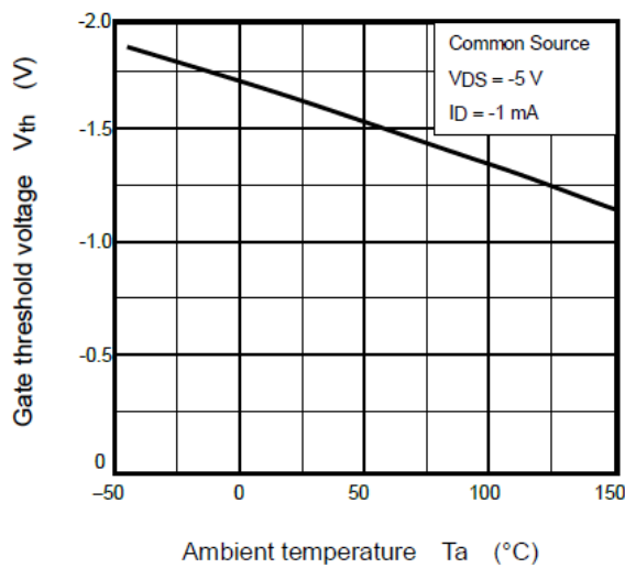
Fig. 7.6 V_{th} - T_a
