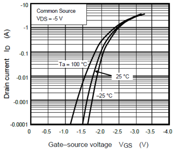
Fig. 7.2 I_D - V_{GS}
