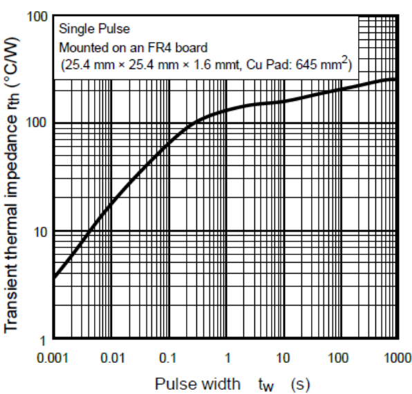
Fig. 7.12 r_{th} - t_w
