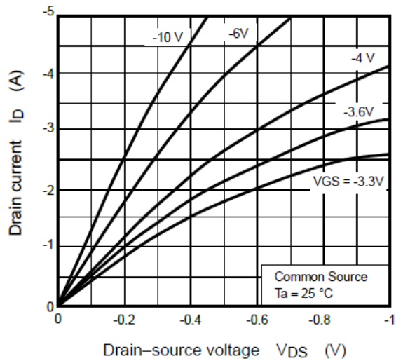
Fig. 7.1 I_D - V_{DS}
