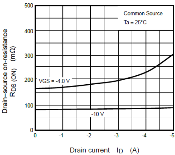
Fig. 7.4 R_{DS(ON)} - I_D
