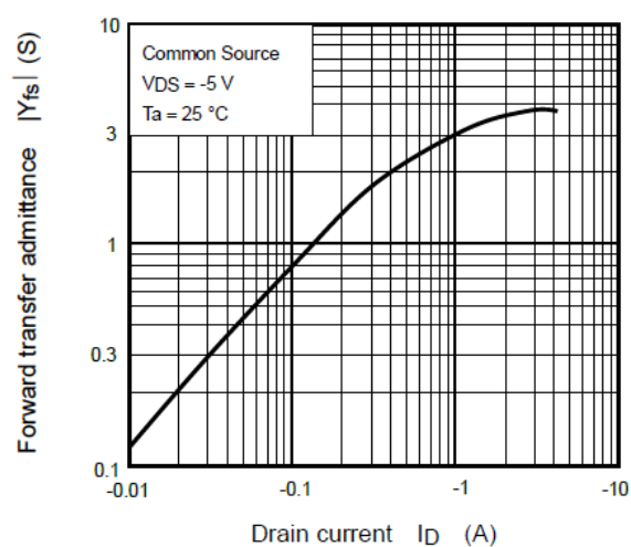
Fig. 7.7 |Y_{fs}| - I_D
