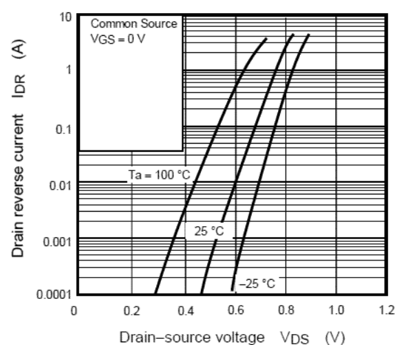
Fig. 7.8 I_{DR} - V_{DS}
