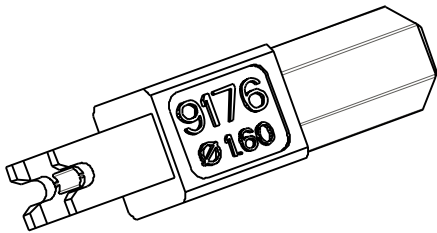
06-9176-7019-02-000 06-9176-7020-02-000 1.6Ø WIRE
