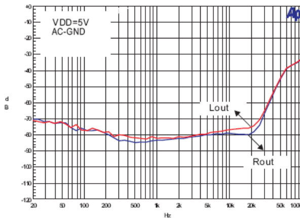
16. PSRR
