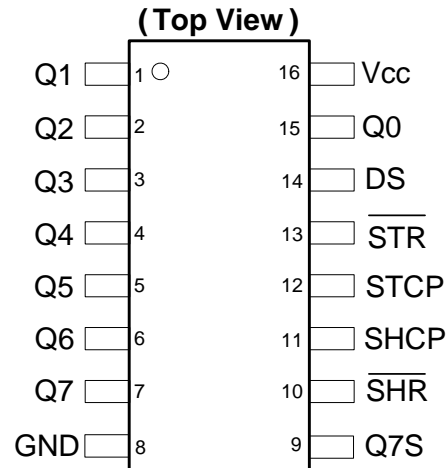
SO-16 / TSSOP-16
