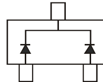
BAT54CW
