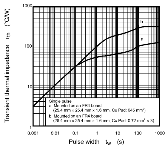
Fig. 8.11 r_{th} - t_w
