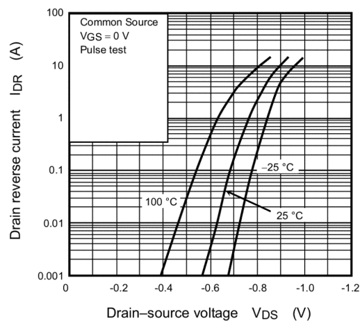
Fig. 8.7 I_{DR} - V_{DS}
