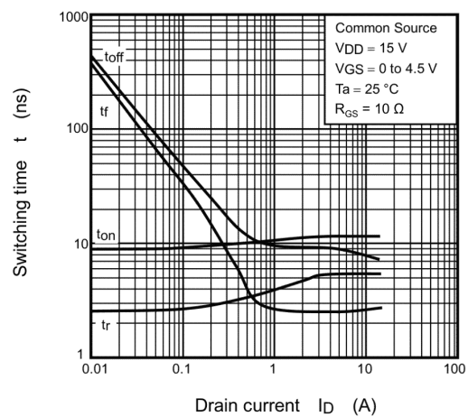
Fig. 8.9 t - I_D
