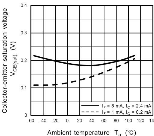
Fig. 11.10 V_{CE(\text{sat})} - T_a
