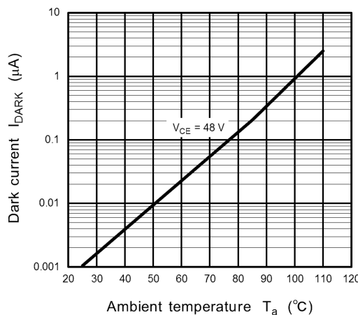
Fig. 11.9 I_{\text{DARK}} - T_a
