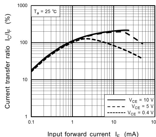
Fig. 11.12 I_C/I_F - I_F
