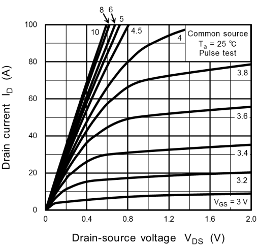
Fig. 8.2 ID - VDS
