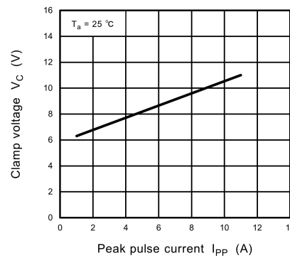
Fig. 10.3.2 V_C - I_{PP}
