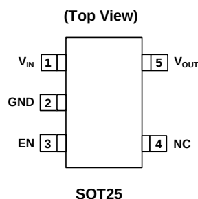
SOT25
