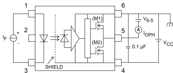
Fig. 13.1.1 I OPH Test Circuit
