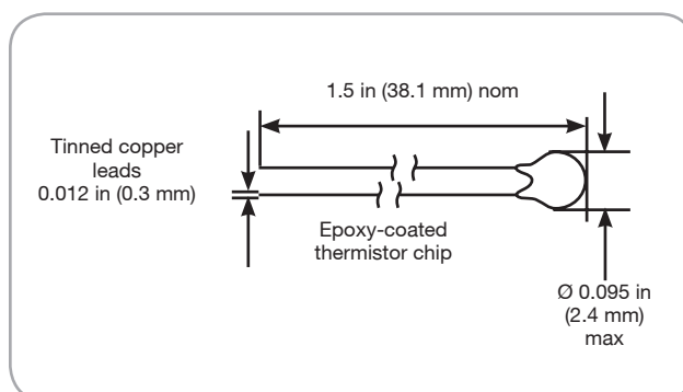
Type DC95 Dimensions
