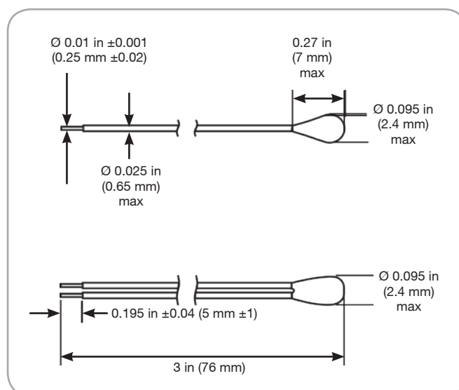
Type TK95 Dimensions
