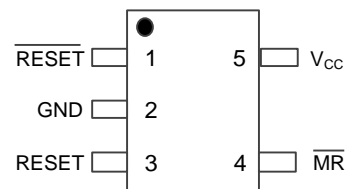
SOT25/SOT353 (PT7M825)
