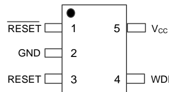
SOT25/SOT353 (PT7M824)
