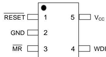
SOT25/SOT353 (PT7M823)
