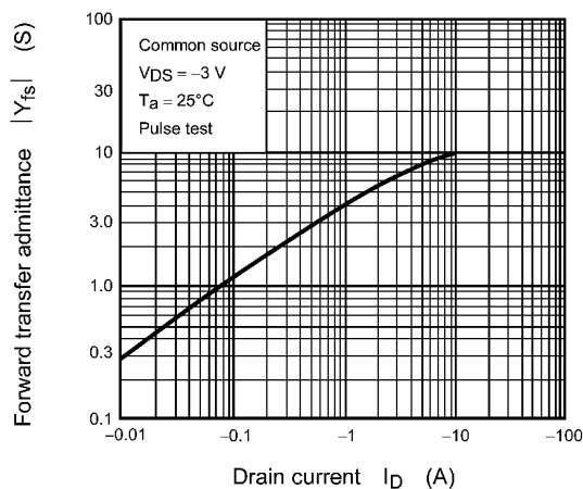
Fig. 7.8 |Y_{fs}| - I_D
