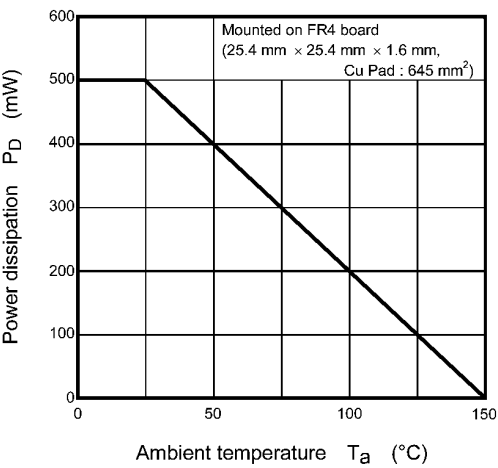
Fig. 7.14 P_D - T_a
