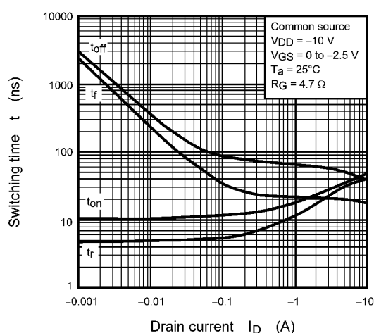
Fig. 7.11 t - I_D
