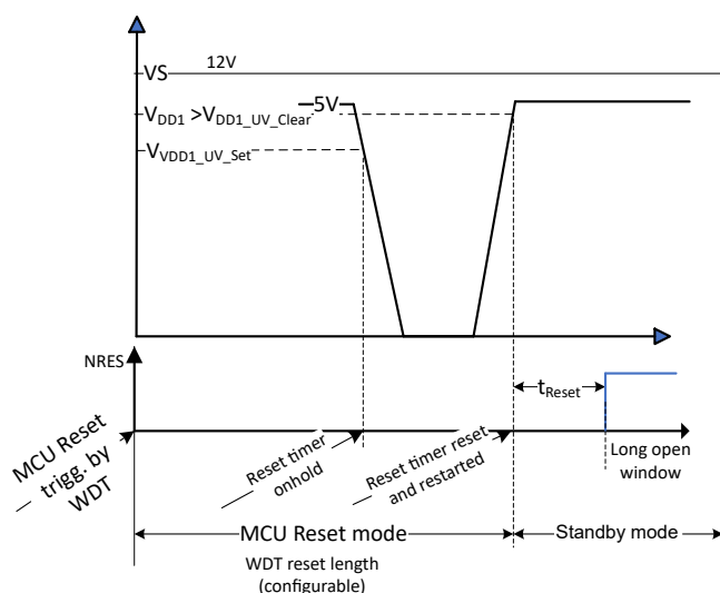
Figure 5-4. VDD1 undervoltage ( V_{DD1} < V_{DD1\_UV\_Set} ) in the MCU Reset mode, RSTLVL = '1', ATA6847-5050
