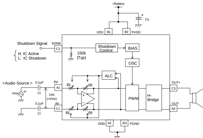
【single end input】
