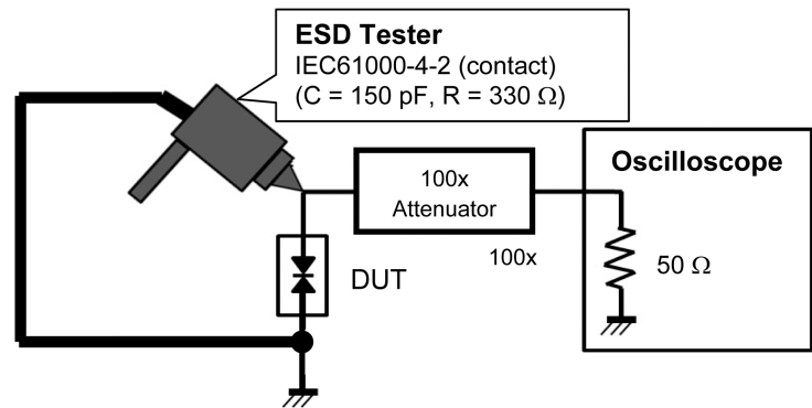
Fig. 6.1.3 IEC61000-4-2 (Contact)
